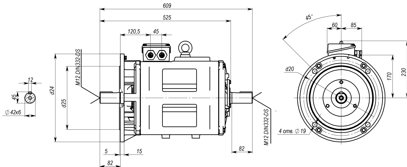
Габаритный чертёж IM 3001; 3002 Dimension drawing IM 3001; 3002
