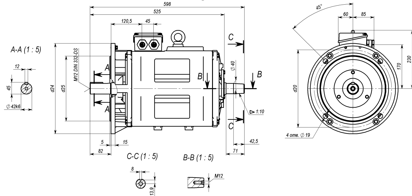
Габаритный чертёж IM 3009 (B5) Dimension drawing IM 3009 (B5)
